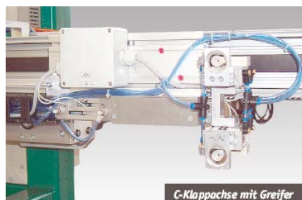
C-Klappachse mit Greifer
