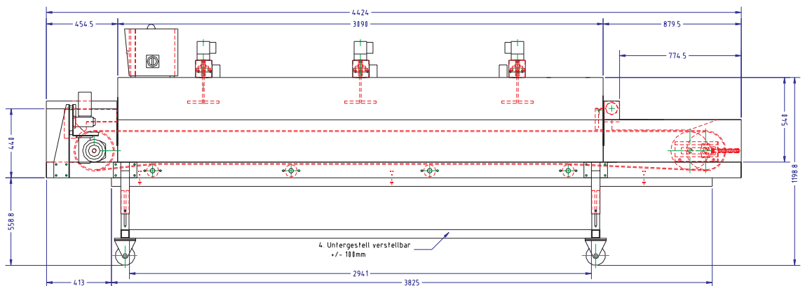
Bild 1 Seitenansicht
