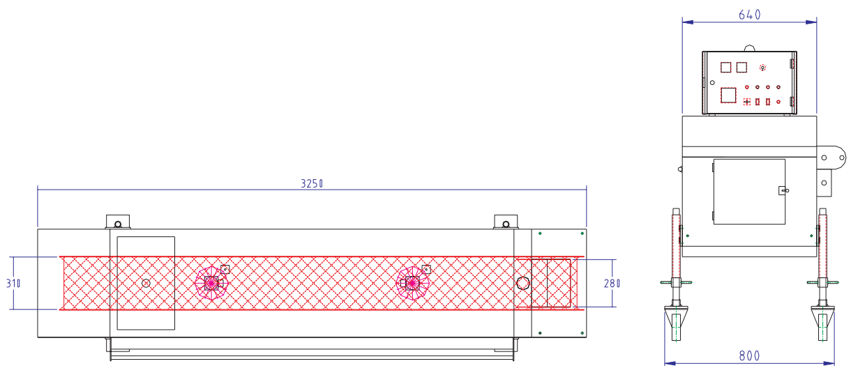
Bild 2 Draufsicht
