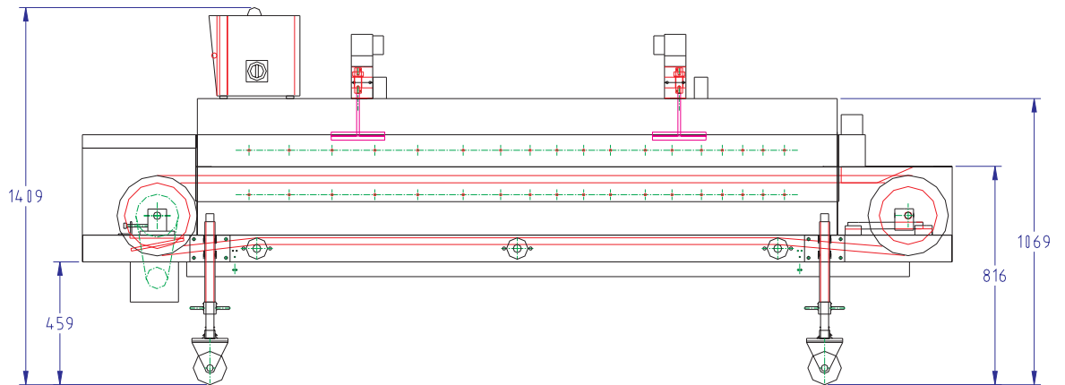
Bild 1 Seitenansicht
