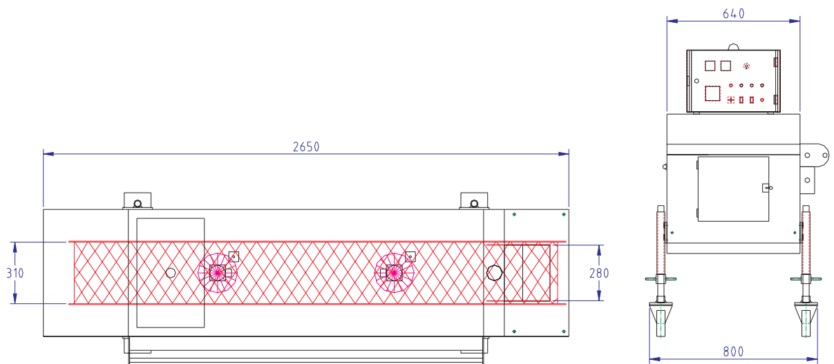
Bild 2 Draufsicht
