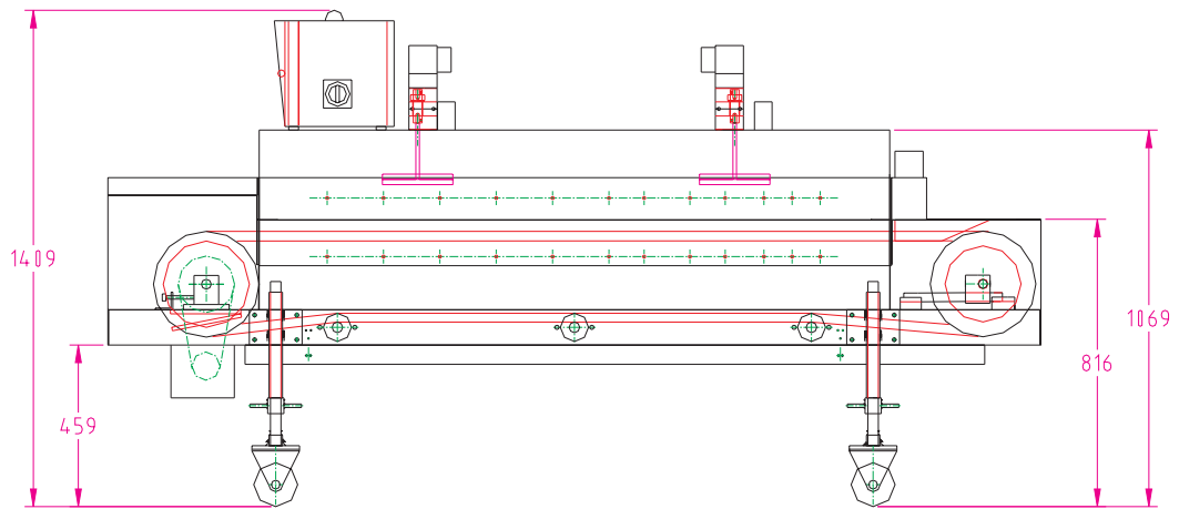
Bild 1 Seitenansicht
